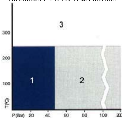
DIAGRAMA PRESIÓN-TEMPERATURA
