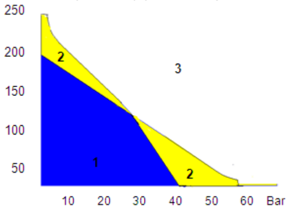
DIAGRAMA PRESION-TEMPERATURA
